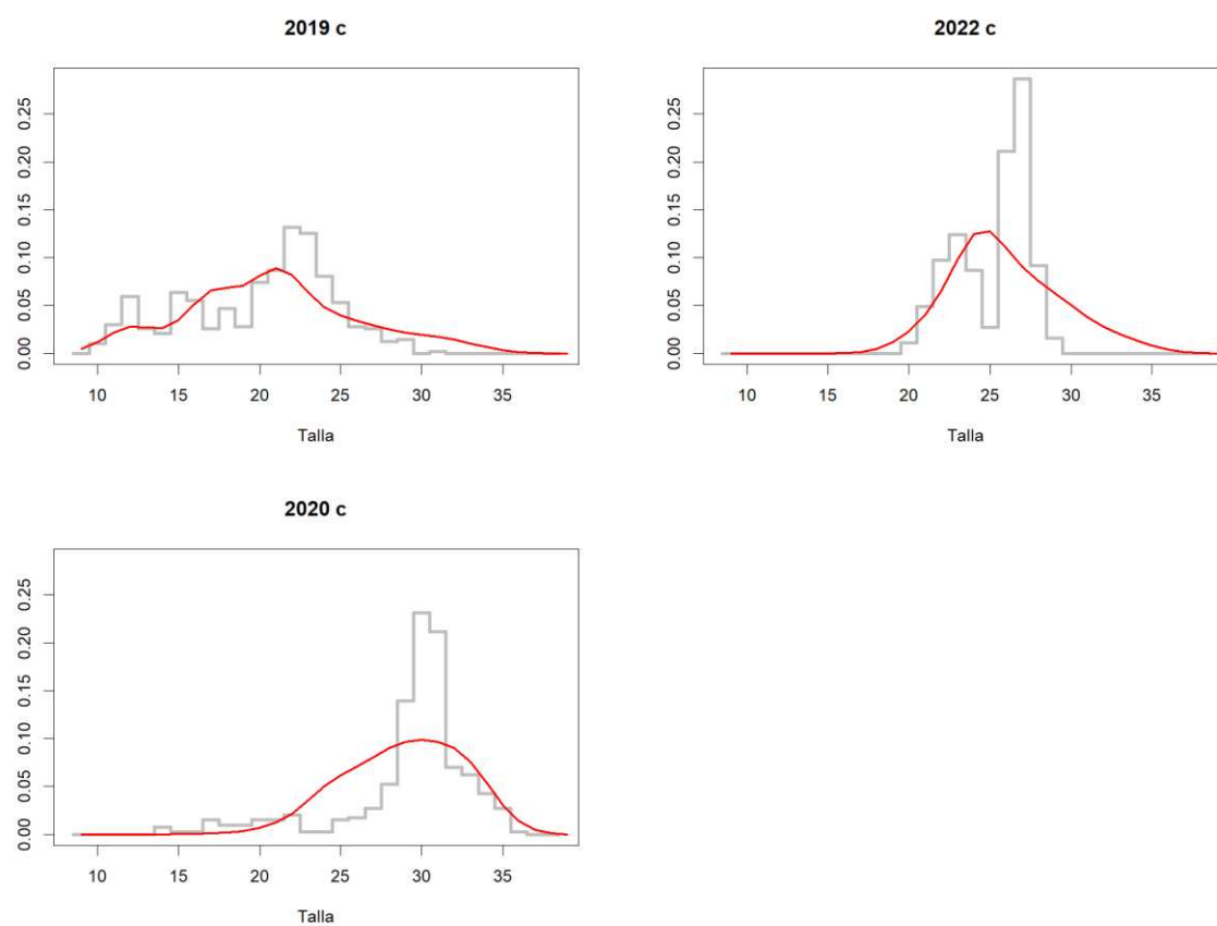
Figura M12. Ajuste del modelo a las composiciones de tallas de los cruceros de Macarela.
