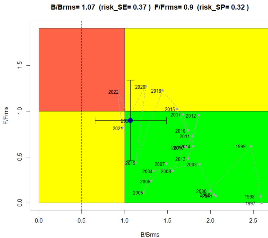
Figura B19. Diagrama de Kobe en botella.
