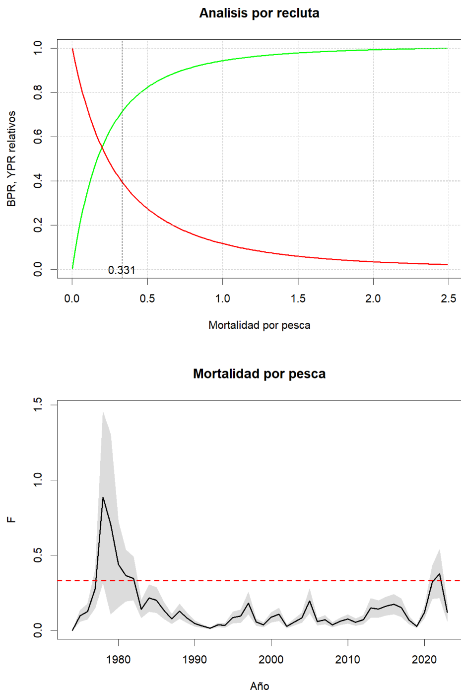
Figura M17. Curvas de equilibrio de rendimiento y biomasa por recluta, mortalidad de referencia en el MSY y mortalidad por pesca anual
