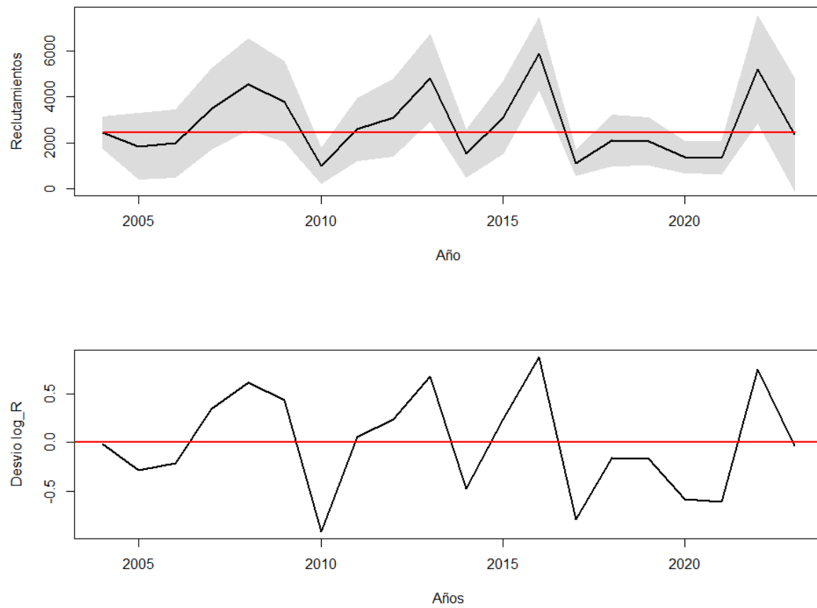
Figura PIC16. Reclutamientos anuales-anuales y anomalía de sus desviaciones en Picudillo.
