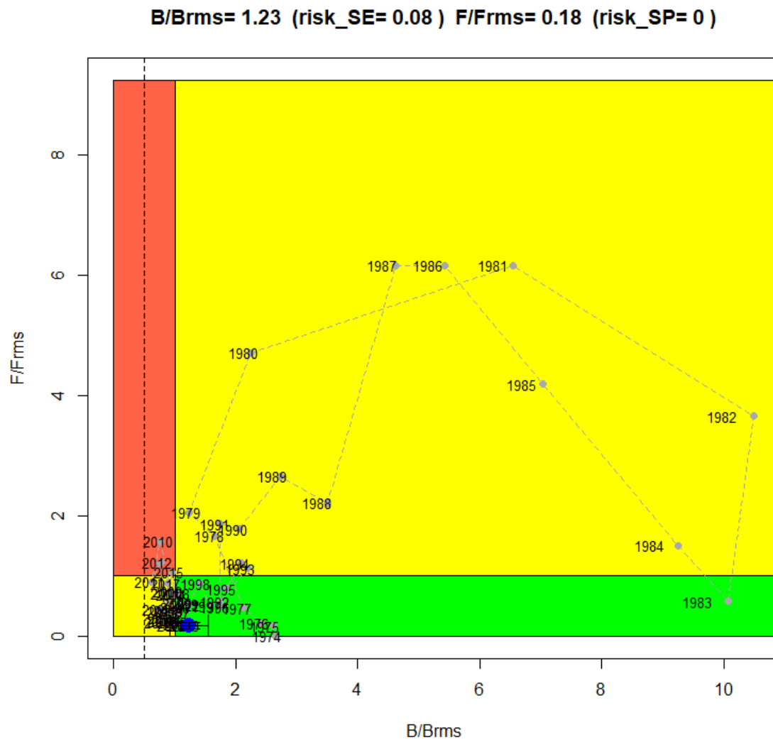
Figura P19. Diagrama de Kobe en Pinchagua.
