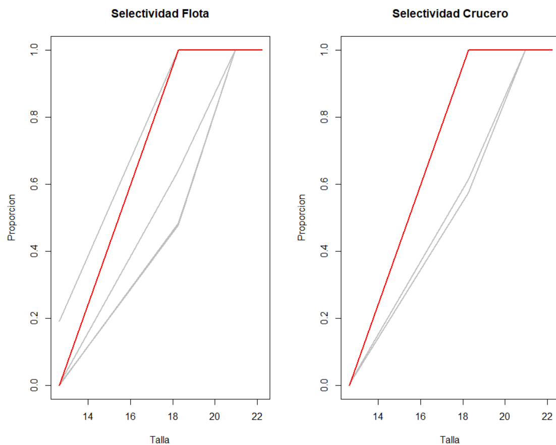
Figura PIC14. Selectividad (líneas grises) de la flota y cruceros acústicos, y proporción de madurez a la talla (línea roja) en Picudillo.
