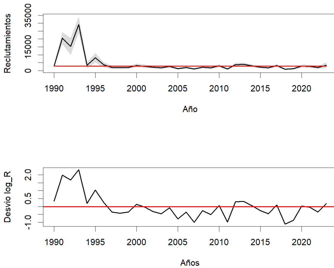
Figura SR 16. Reclutamientos anuales-anuales y anomalía de sus deviaciones en Sardina Redonda.
