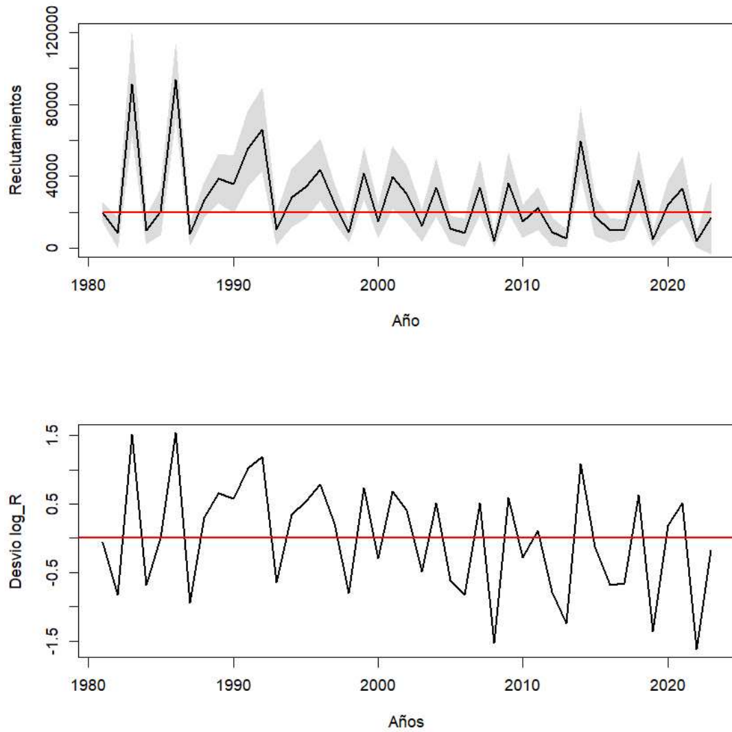
Figura CHC16. Reclutamientos anuales-anuales y anomalía de sus desviaciones en Chihuahua.
