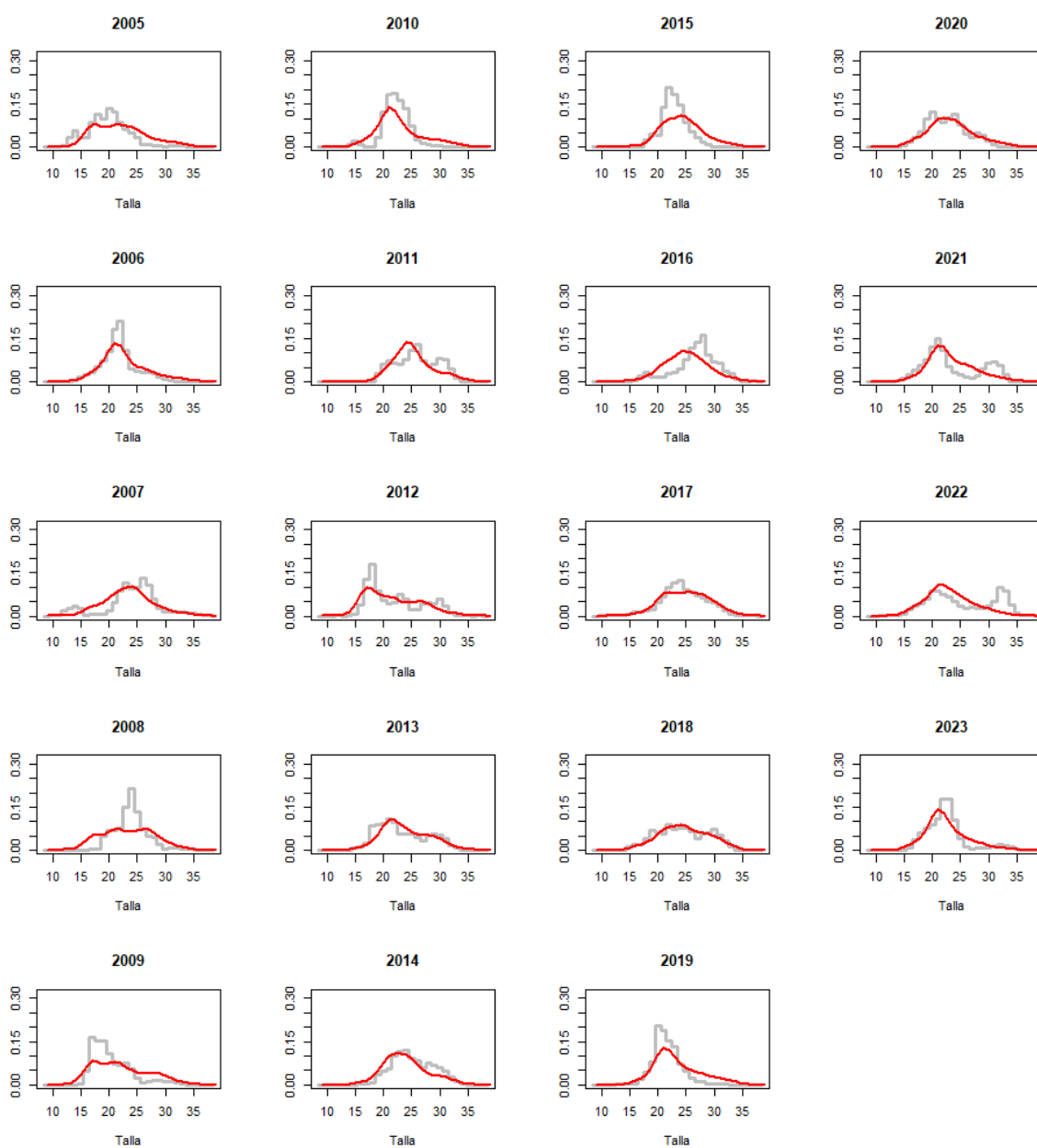
Figura M11. (continuación)
