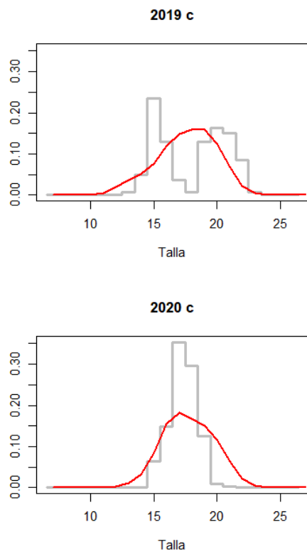
Figura CHC12. Ajuste del modelo a las composiciones de tallas de los cruceros de Chuhueco
