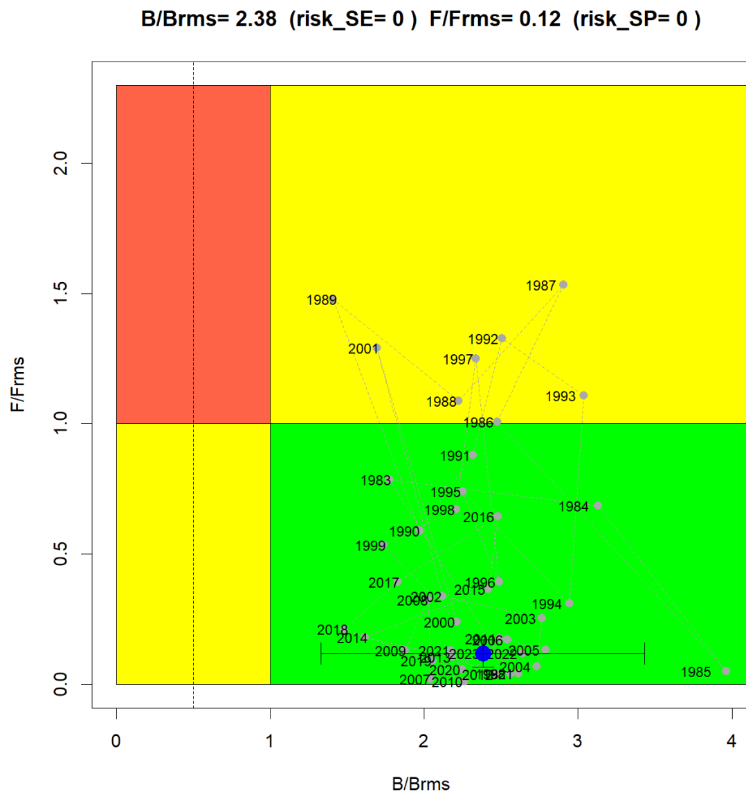
Figura CH19. Diagrama de Kobe en Chuhueco.
